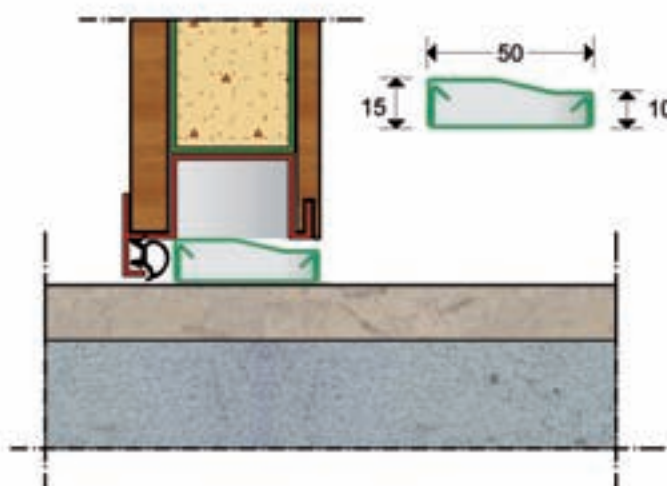
SEZIONE VERTICALE PORTA con soglia a battuta INOX Sat.
