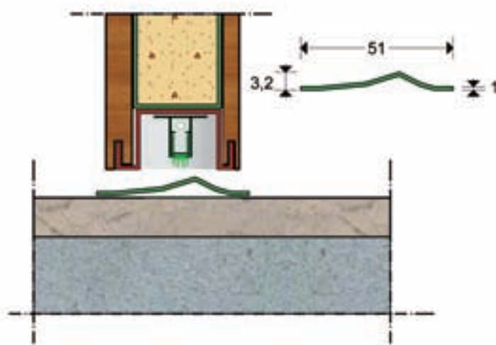
SEZIONE VERTICALE PORTA con soglia a battuta Slim INOX Sat.
