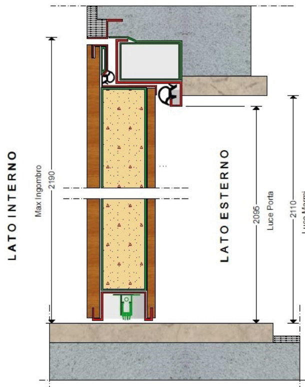
SEZIONE VERTICALE PORTA
