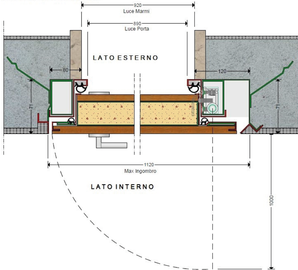
SEZIONE ORIZZONTALE PORTA
